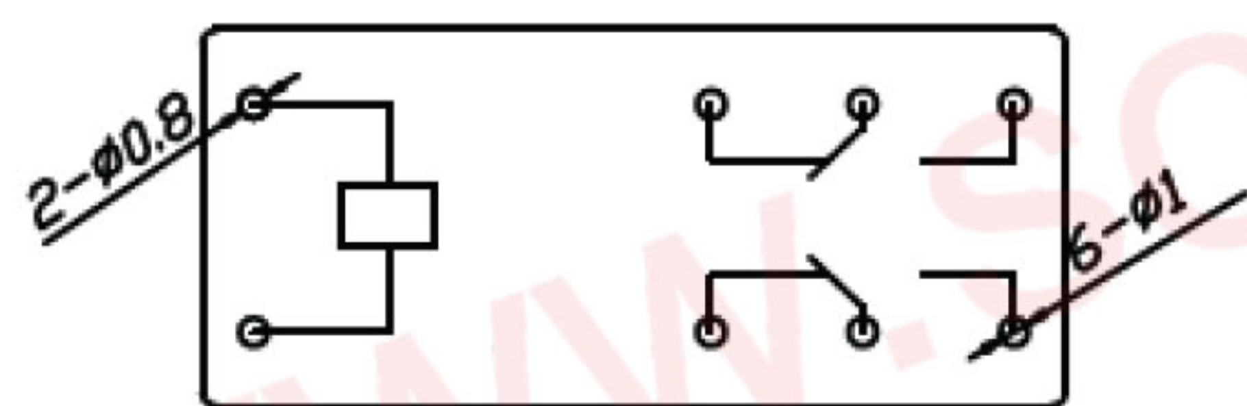
电气原理图
