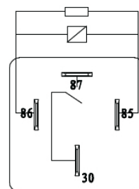
常开 A 型
