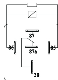
转换 C 型
