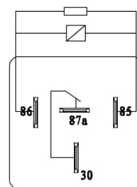
常闭 B 型
