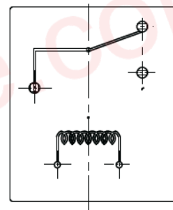
PCB板示意图 (底视图)
